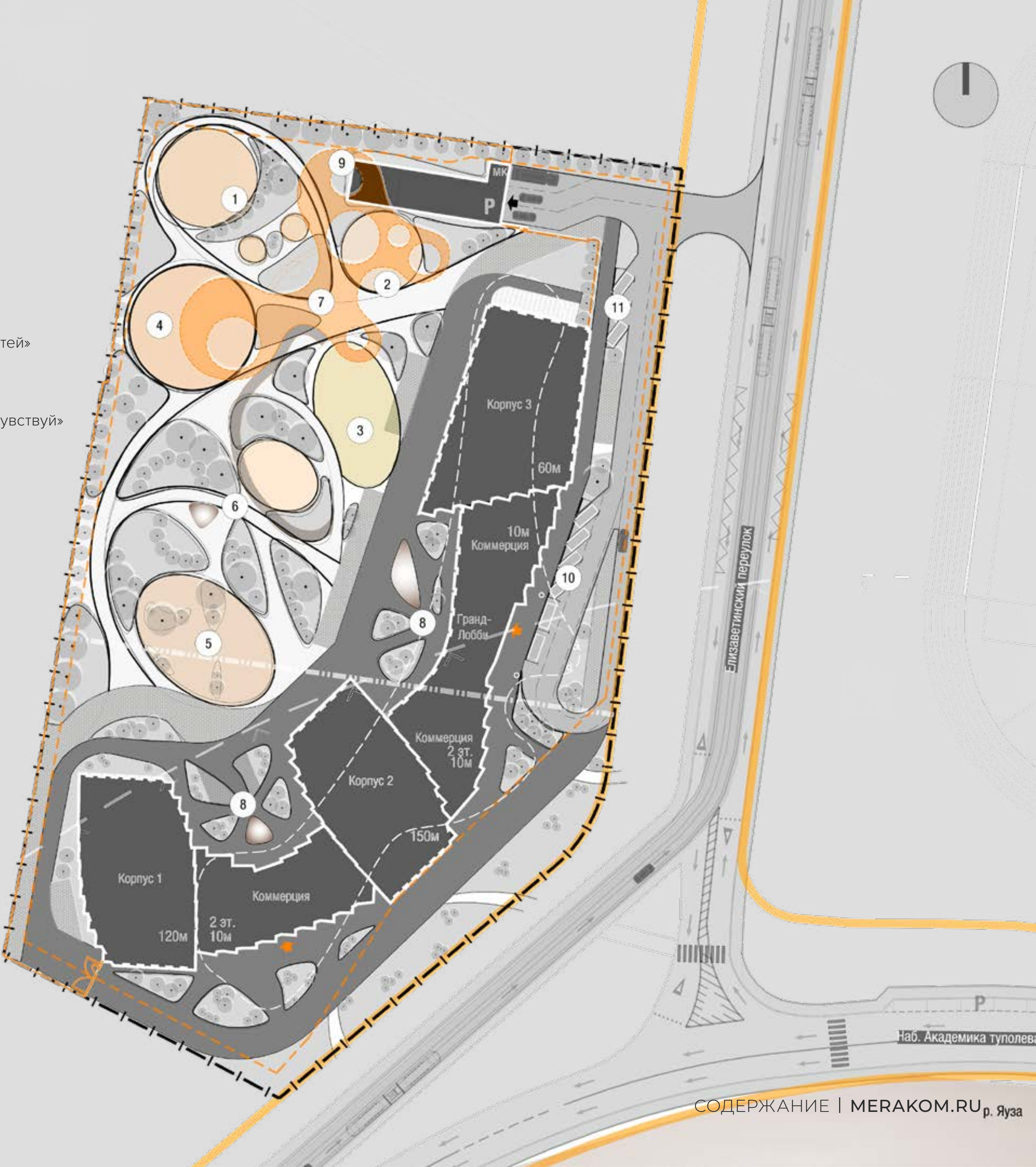
Генеральный план
