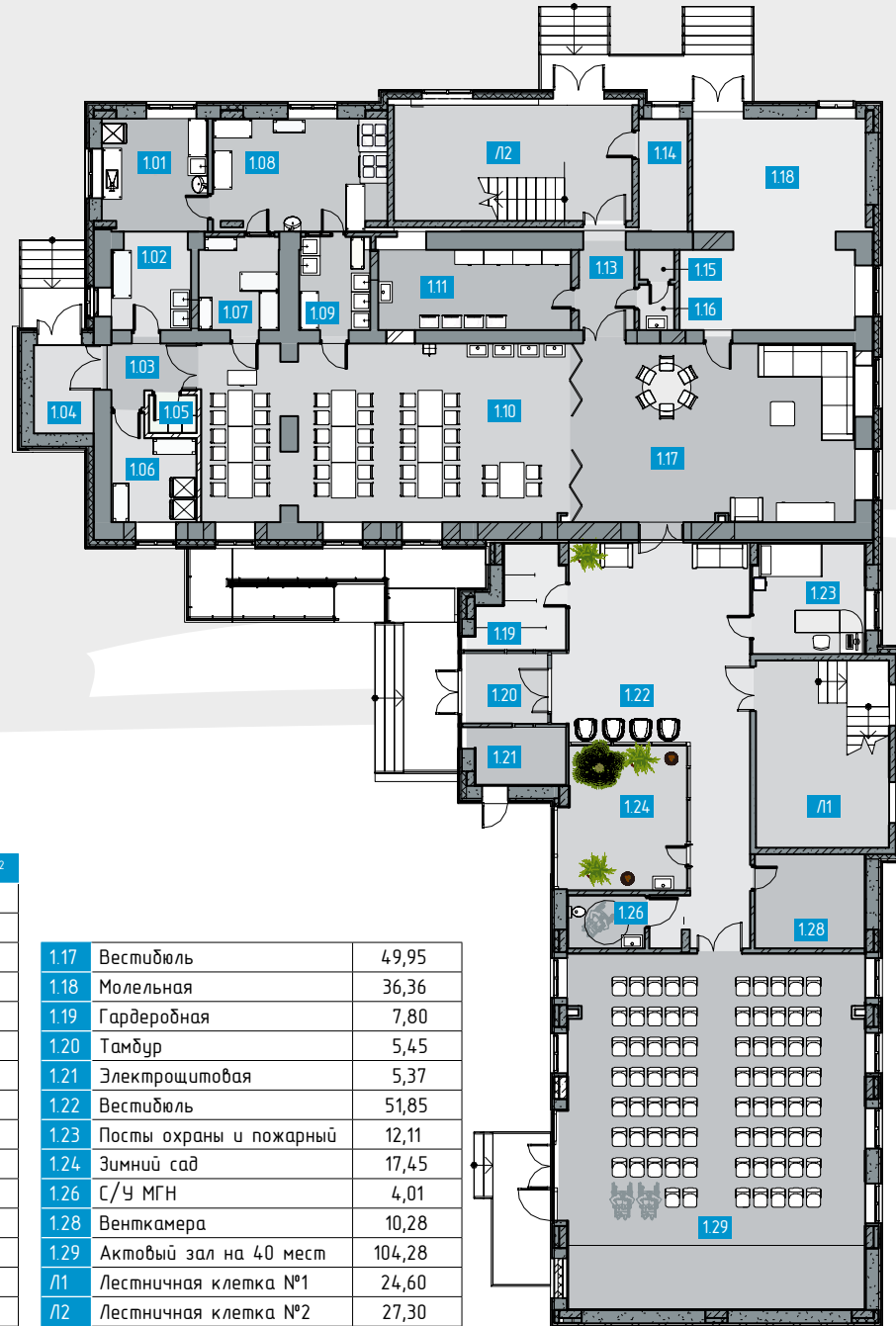
Экпликация помещений 1-го этажа
