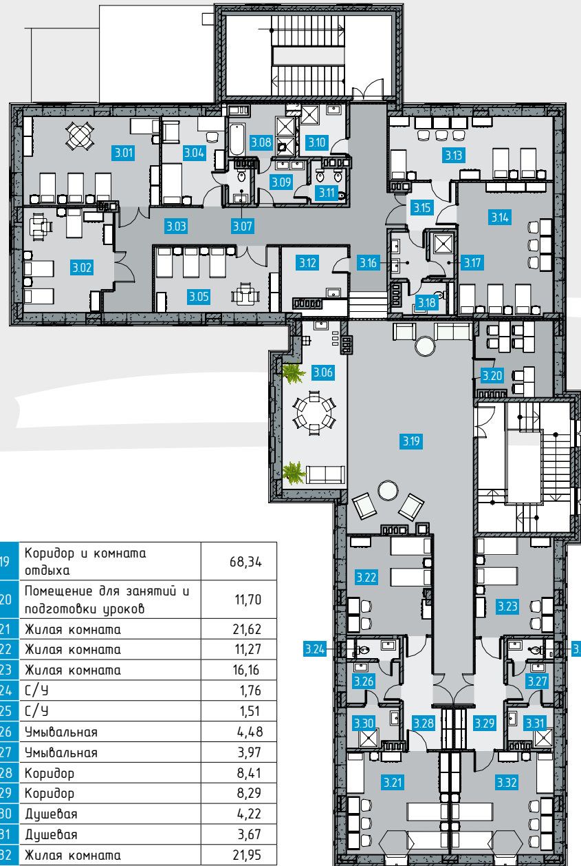
Экспликация помещений 3-го этажа
